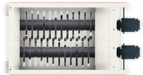
Schneidisch 12 Messer
